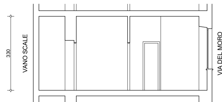
SEZIONE S-S' POST OPERAM rapp. 1:100
