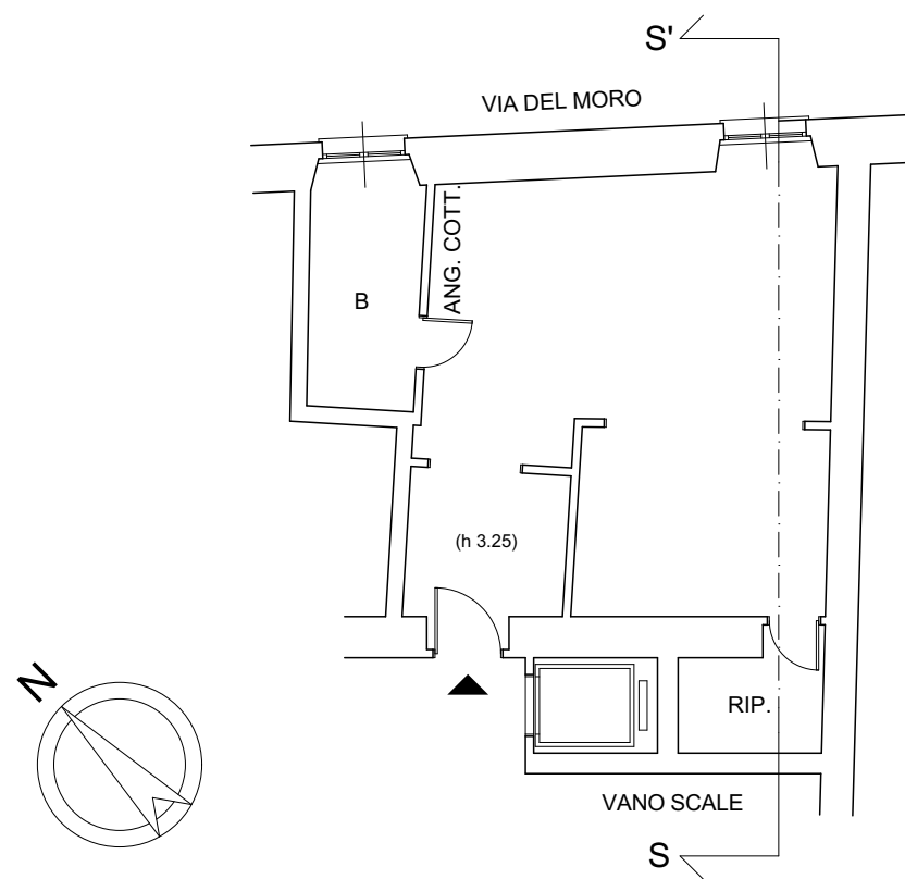
PLANIMETRIA ANTE OPERAM rapp. 1:100
