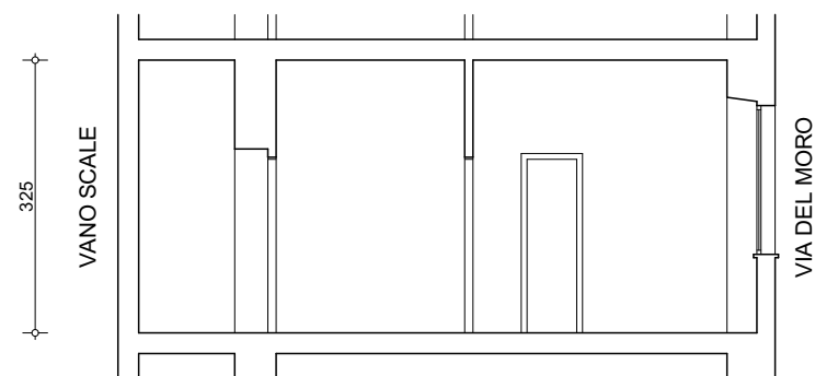
SEZIONE S-S' ANTE OPERAM rapp. 1:100
